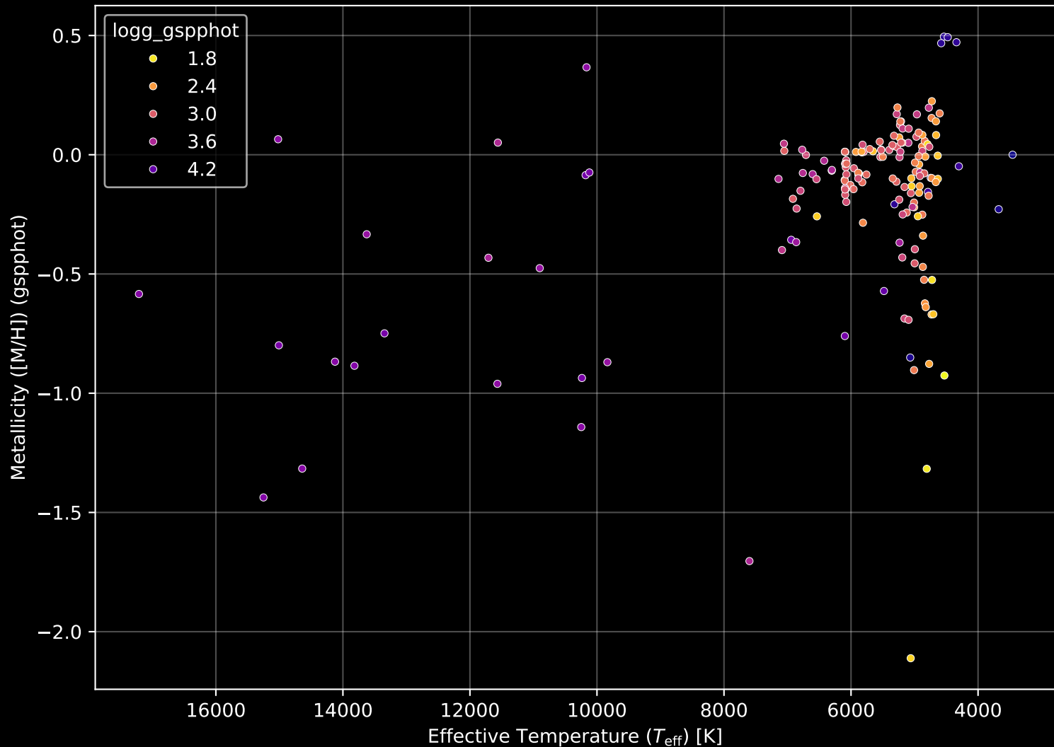
APOGEE DR17 Field: [139+04] Stellar Population Parameters (n= 171)
